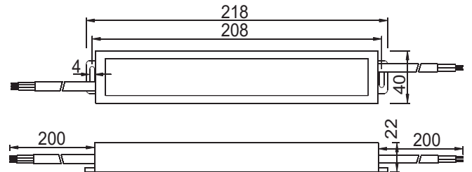
Schéma technique
