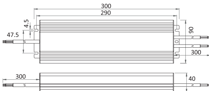
Schémas techniques
