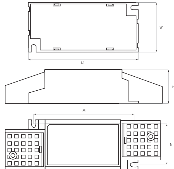
Schéma technique
