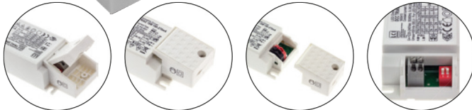
Serre-câble amovible
