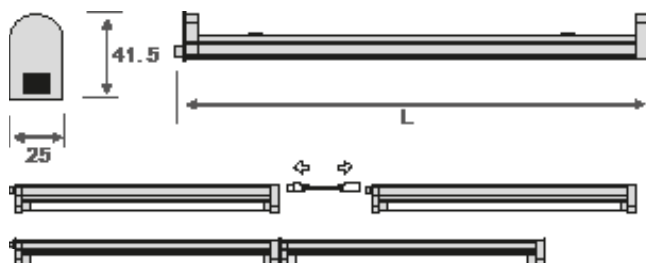
Schéma technique
