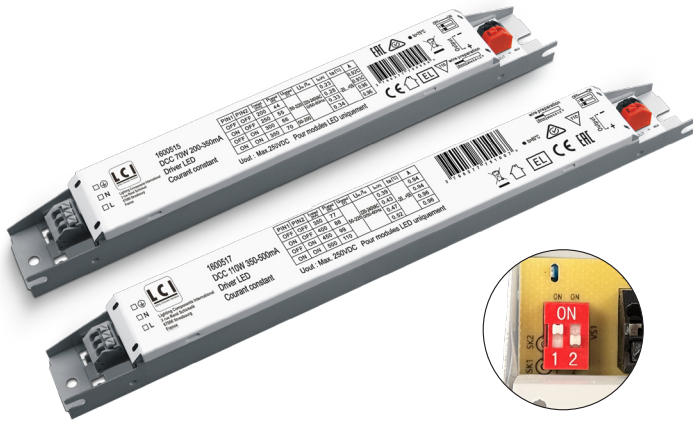
DIP switches Réglage courant
