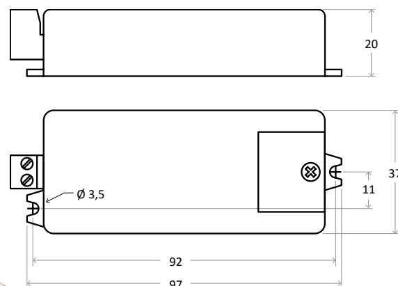
Schéma technique
