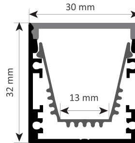
Schéma technique
