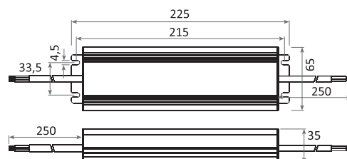
Schémas techniques
