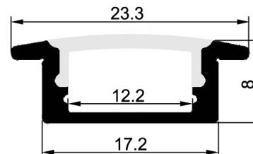
Schéma technique
