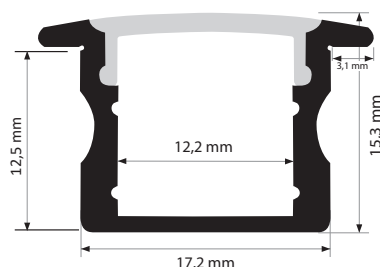
Schéma technique
