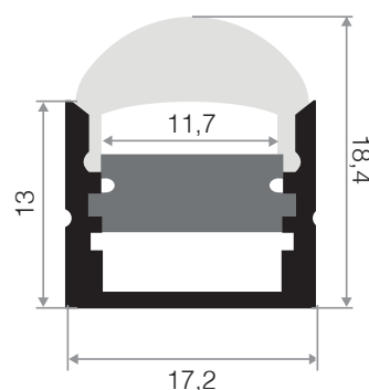
Schéma technique
