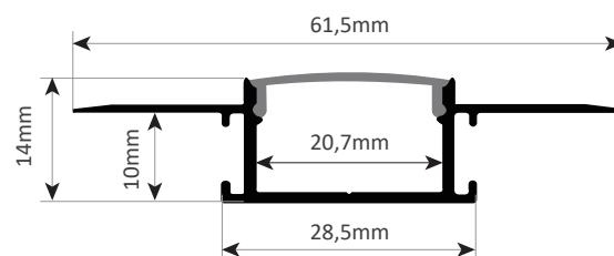
Schéma technique
