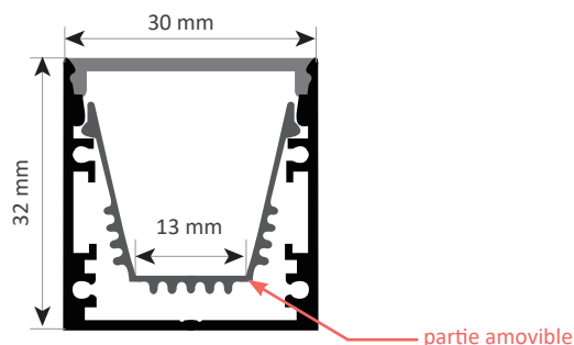
Schéma technique
