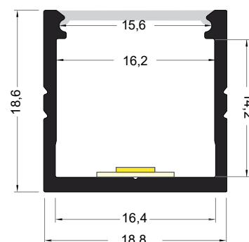
Schéma technique
